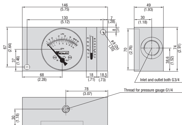
Dimensions SDM-750
